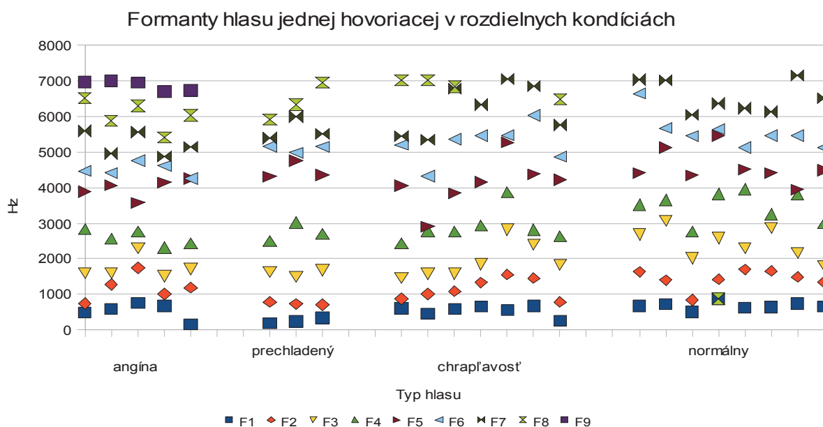
Graf 2: Hodnoty formantov jednej hovoriacej počas angíny, zachrípnutia, zdravý hlas a hlas počas prechladenia
