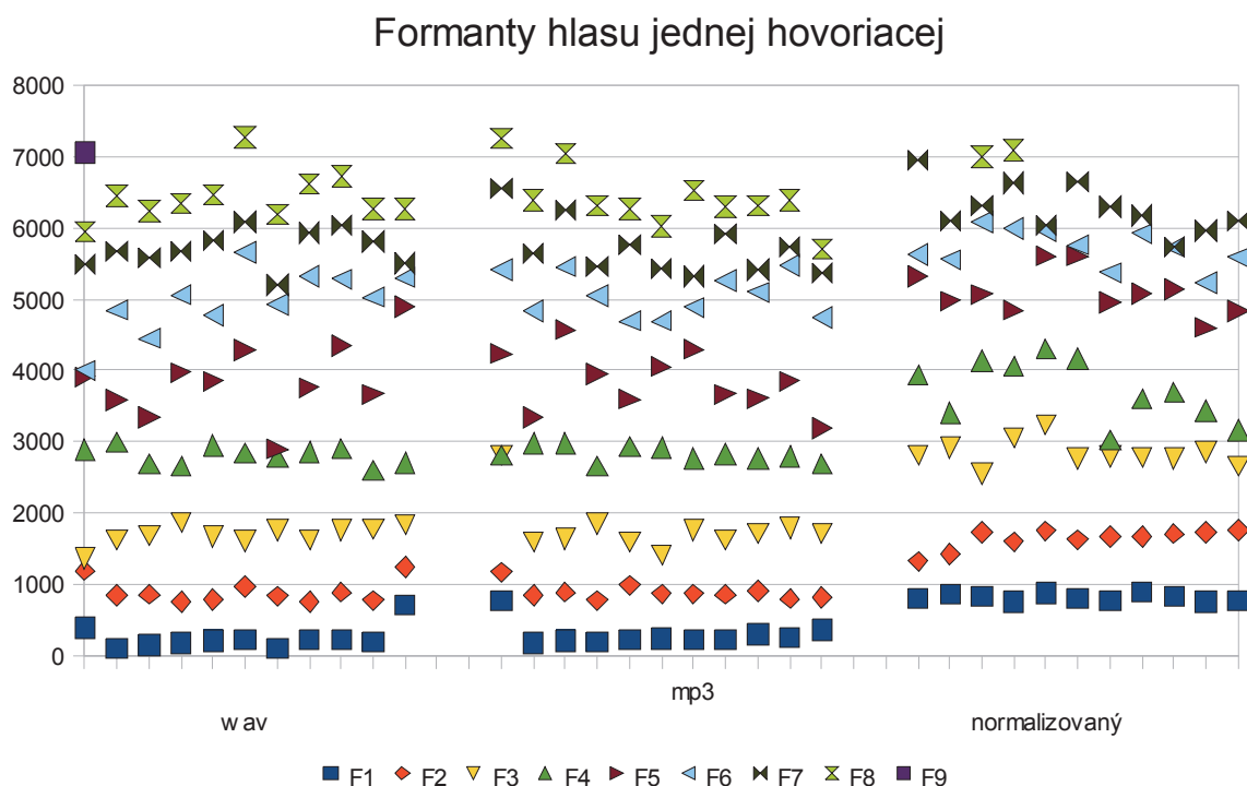
Graf 1: Hodnoty formantov vokálu a jednej hovoriacej v totožnej nahrávke vo formáte wav , mp3 a normalizovanej nahrávky
