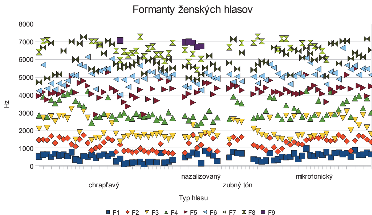
Graf 5: Hodnoty formantov rôznych ženských hlasov
