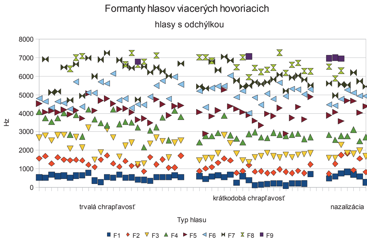
Graf 3: Hodnoty formantov hlasov tvorených poškodenými hlasivkami v porovnaní s hlasom tvoreným zdravými hlasivkami
