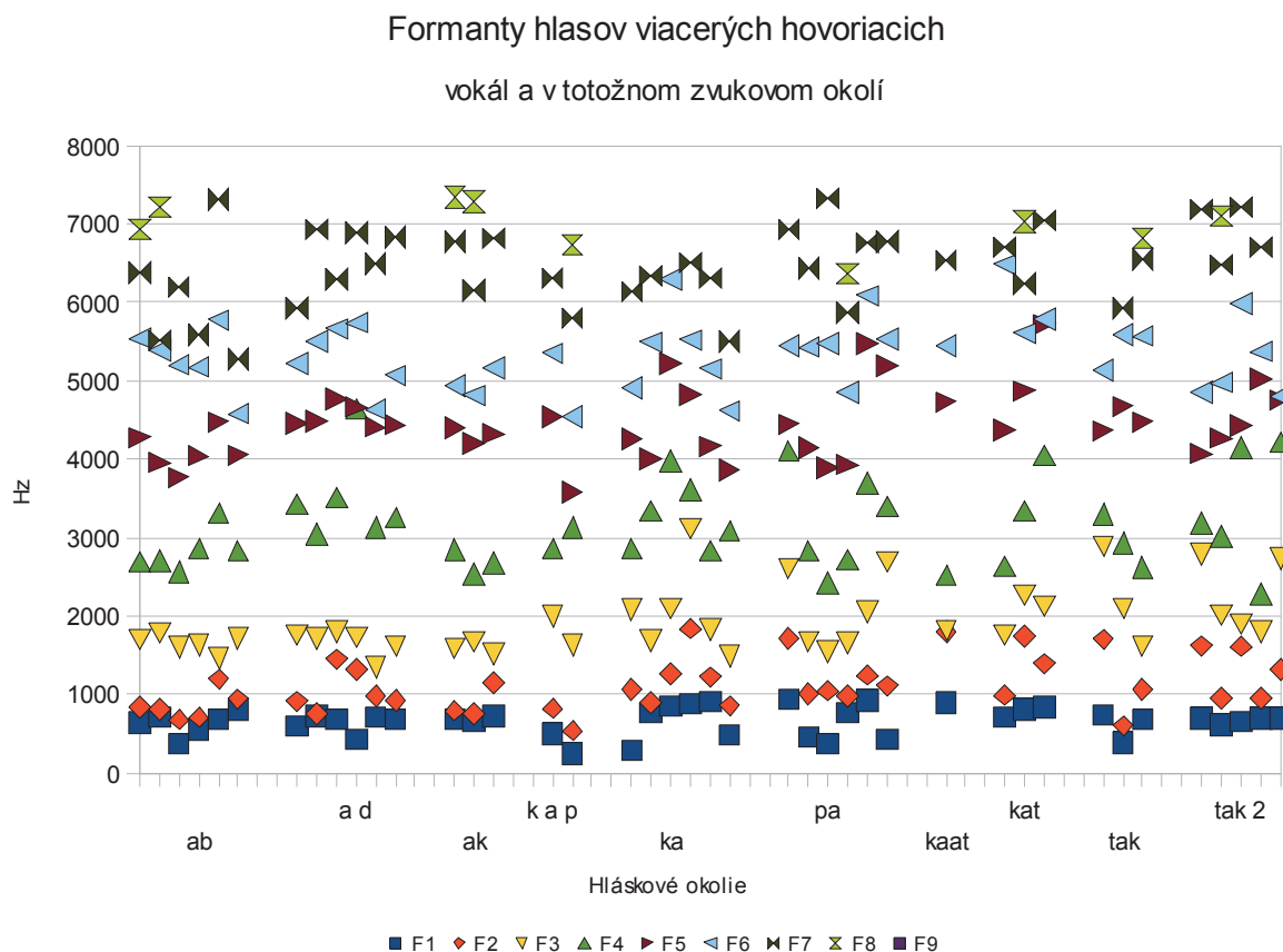
Graf 4: Zobrazenie hodnôt formantov vokálu a viacerých hovoriacich v totožnom zvukovom okolí
