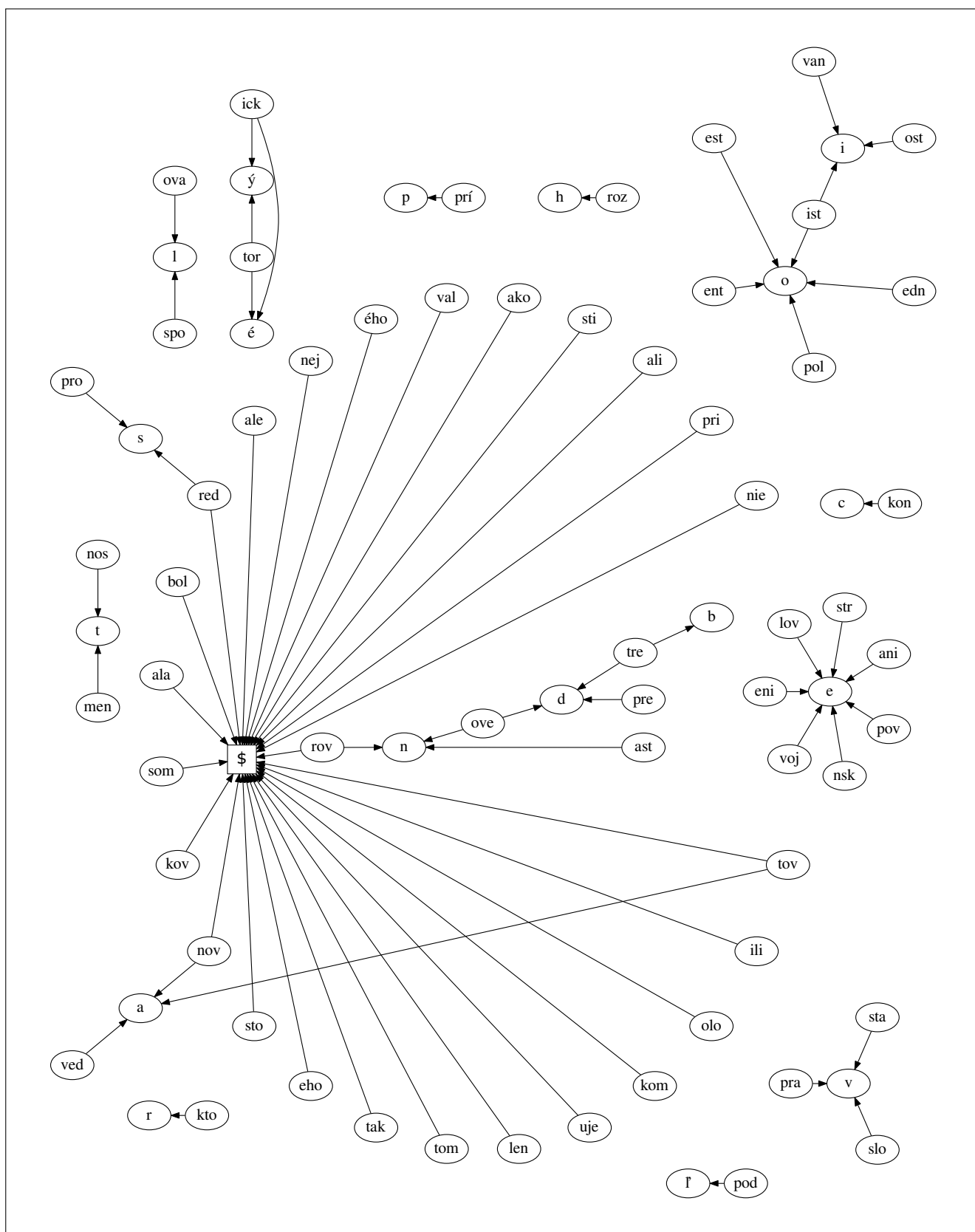
Obr. 6: Znázornenie prográdnych prechodov medzi trigramom a unigramom v rámci slov. Zobrazené sú iba najčastejšie trigramy a prechody. Symbolom $ je označený koniec slova.
