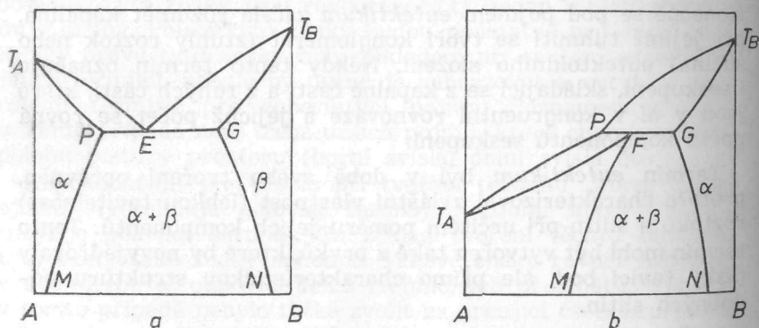
Obr. 2. Diagramy rovnováhy dvojnásobného seskupení s omezenou vzájemnou rozpustitelností složek v tuhém skupenství a – eutektikum; b – peritektikum
