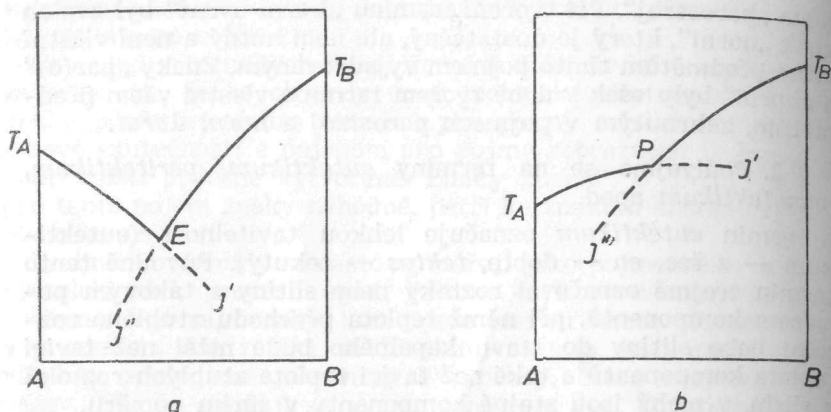
Obr. 1. Diagramy kapaliny dvojího seskupení s omezenou vzájemnou rozpustitelností složek v tuhém skupenství a – eutektikum; b – peritektikum
